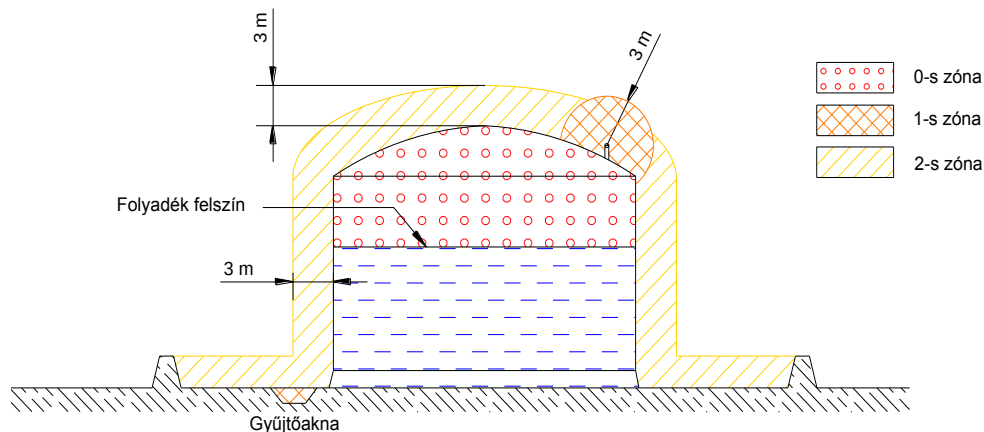
1. Rajz Belső úszótető nélküli merevített tartály, szabadtéren elhelyezve
