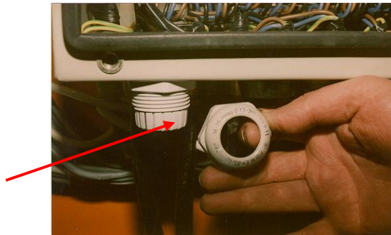
Rögzítő körmök (tömítő gumi gyűrűvel együtt szorítva)
