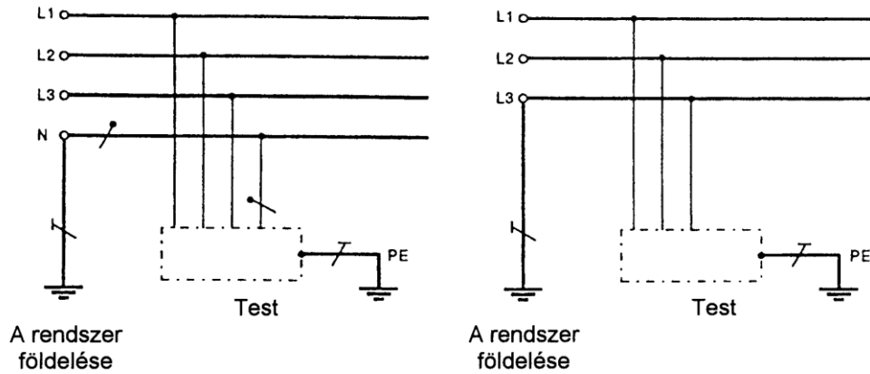
TT-rendszer
